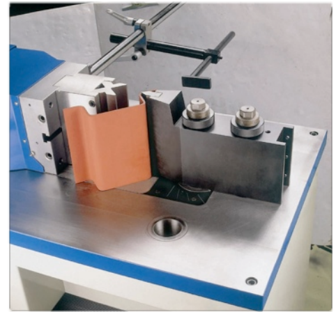
Multi-Vee Press Brake
