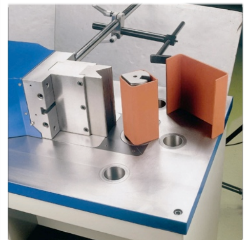
Single-Vee Press Brake
